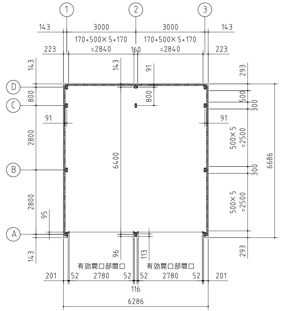
平面図
